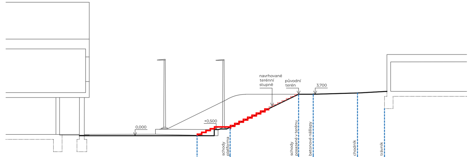
Řez AA'
